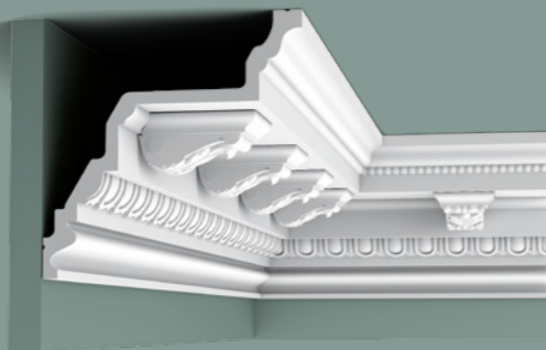
1 C307 + C307A 2 C307A: 7,5 x 4 x 9,4 cm Duropolymer® 19,5 9,4 4 9,4 26,9
