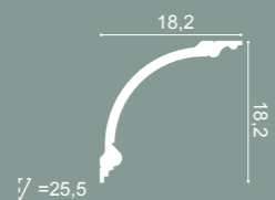
C338 BA'ROCK 200 x 18,2 x 18,2 cm Purotouch ®
