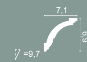
CX101 200 x 6,9 x 7,1 cm Duropolymer®
