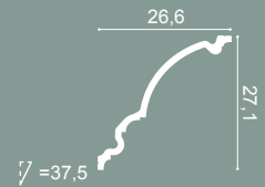
C336 BA'ROCK 200 x 27,1 x 26,6 cm Purotouch ®
