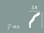
CX112 200 x 5,4 x 3,8 cm Duropolymer®
