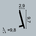
SX179 DIAGONAL 200 x 9,7 x 2,9 cm Duropolymer®
