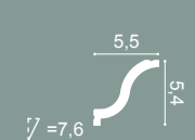
CX108 200 x 5,4 x 5,5 cm Duropolymer®
