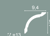
CX129 200 x 9,4 x 9,4 cm Duropolymer®
