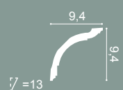
5 CX127 | CX127F 200 x 9,4 x 9,4 cm Duropolymer®
