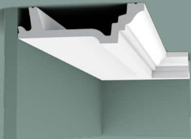
C305 200 x 4,7 x 15,5 cm Purotouch® 15,5 4,7 5,6 ∇ = 15,9
