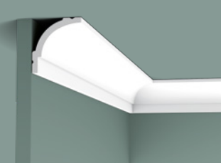
CB525 200 x 6,5 x 6 cm Durofoam®
